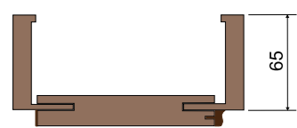
profil zárubně č. 6
