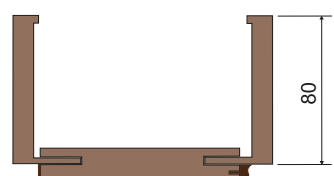
profil zárubně č. 3
