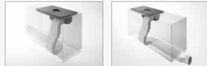
Příklady možného odtahového potrubí v soklu Example of duct-out mode configuration with lateral outlet
